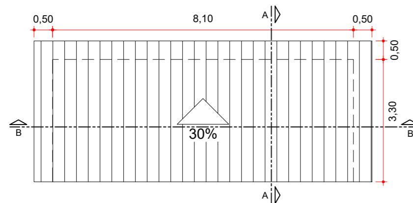
PLANTA DE COBERTURA ESCALA 1:100
