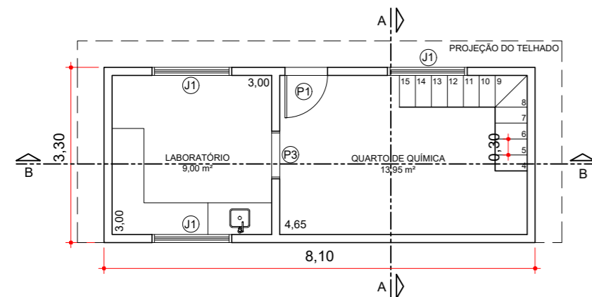
PLANTA BAIXA - PAVIMENTO SUPERIOR ESCALA 1:100
