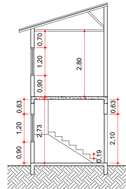
CORTE AA ESCALA 1:100
