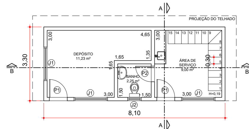
PLANTA BAIXA - PAVIMENTO INFERIOR ESCALA 1:100
