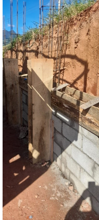
Estrutura de concreto armado pilares e cintas intermediárias
